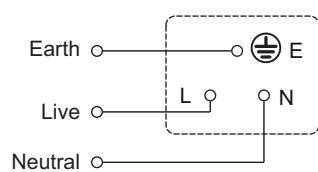
Socket
